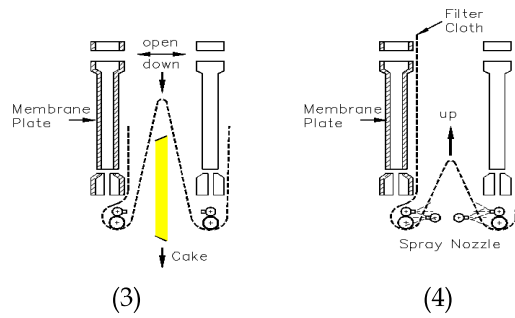
Fig 2 가압탈수기 공정도
