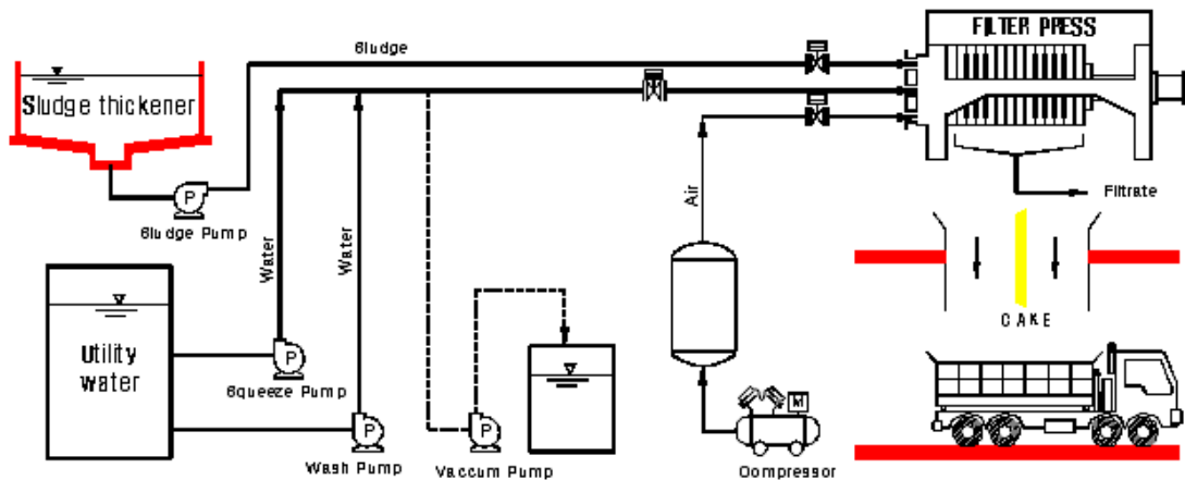
Fig 1 가압탈수기를 적용한 탈수공정
